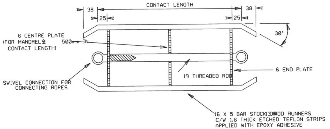
LONGITUDINAL SECTION OF MANDREL
