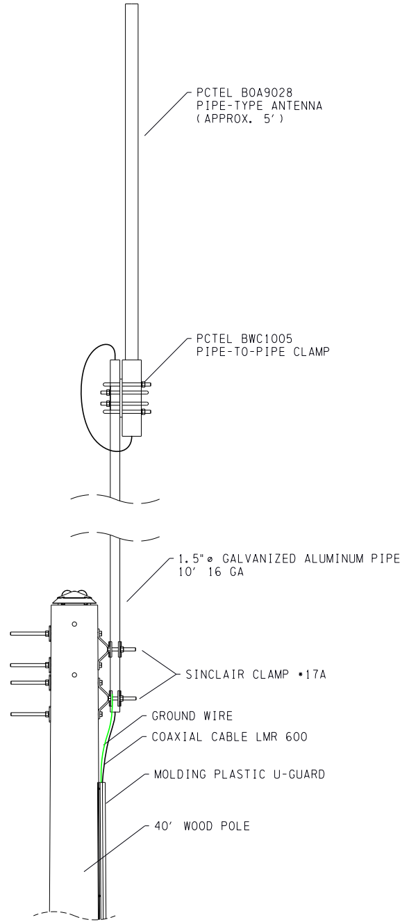
A DETAIL SCALE: N.T.S.
